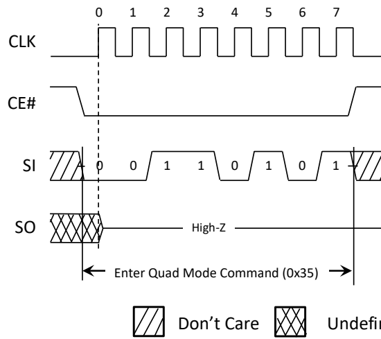
Figure 12 : Quad Mode Enable 0x35
